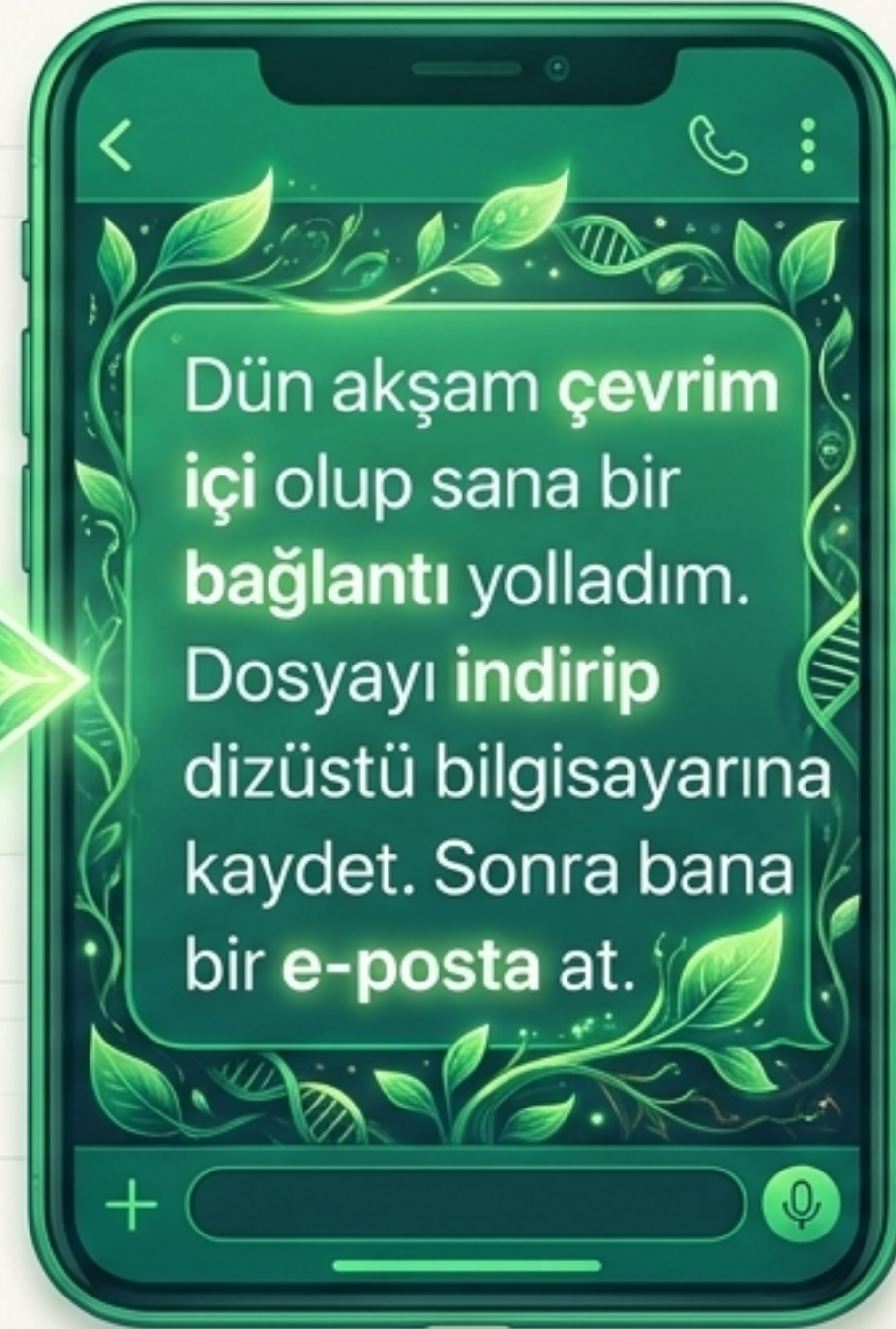
Doğru Metin
