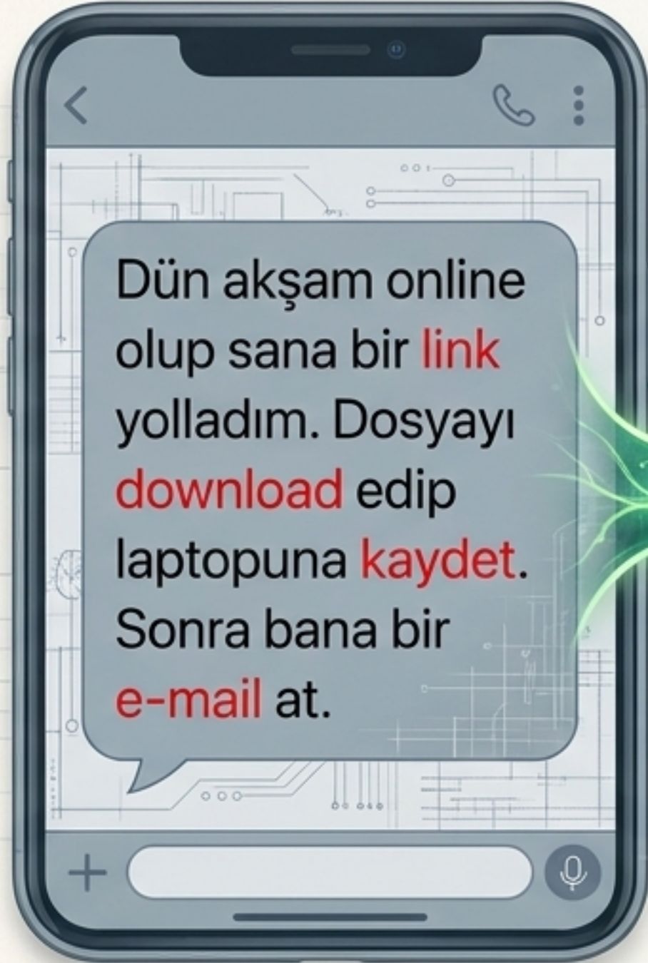
Hatalı Metin
